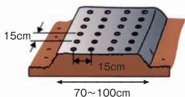
図2 種球の準備
